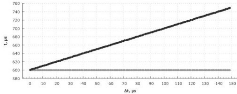
Рисунок 5 - Зависимость оценок времен прихода двух сложных сигналов от разности времени прихода, полученная методом максимального правдоподобия.
