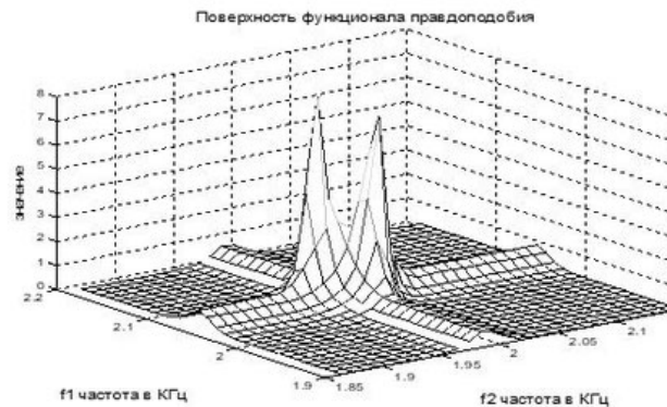
Рисунок 2 - поверхность обратного преобразованного функционала правдоподобия при малом разнесении частот радиопульсов: f_1 = 2 кГц, f_2 = 2,03 кГц. Амплитуды радиопульсов U_1 = 2 , U_2 = 2 , отношение сигнал/шум равно 10 дБ, длительность радиопульсов 25 мс.
