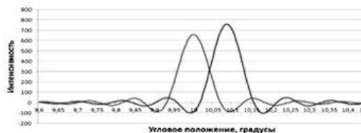
Рисунок 9 - Угловое разрешение интенсивности света от двух лазерных указок. Интенсивности света равны U_1=6.6 , U_2=7.6 , Угловые положения \beta_1=10 градусов, \beta_2=10.084 градуса
